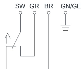
Anschlußschema (ohne Flüssigkeit)
